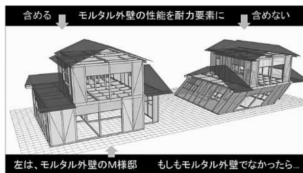
図7 木造住宅倒壊解析 wallstatによるシミュレーション例
